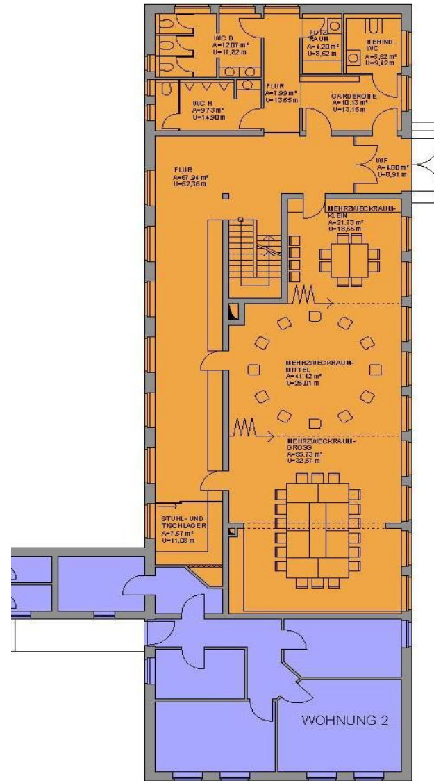
GRUNDRISS EG
