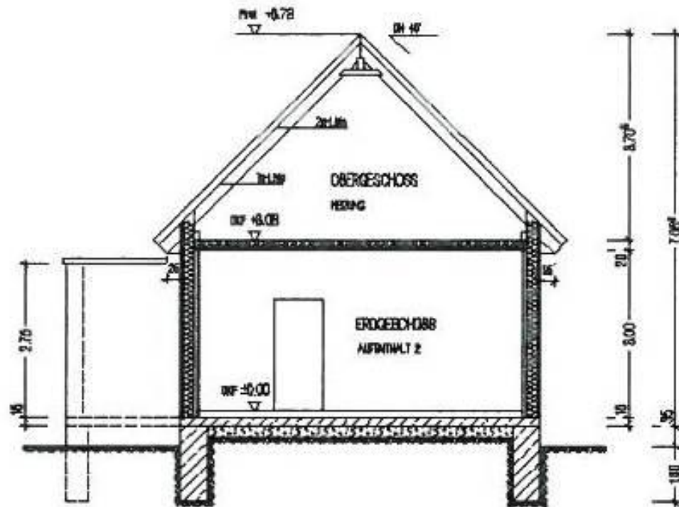
SCHNITT
